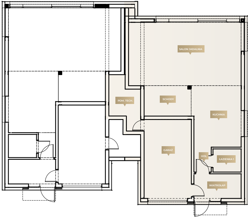
RZUT PARTERU
