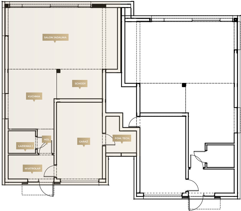
RZUT PARTERU
